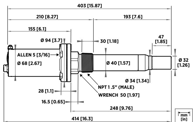
MGP261 dimensions
